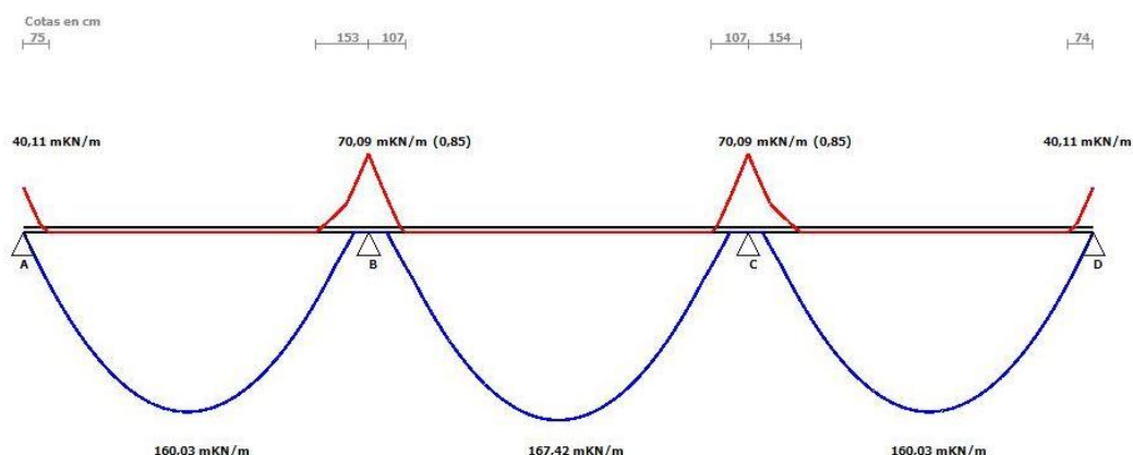
Figura.- Envolvente de flexión
