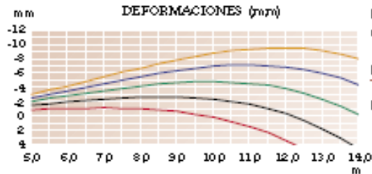
Figura.- Ejemplo de placa alveolar de 35 cm de canto
