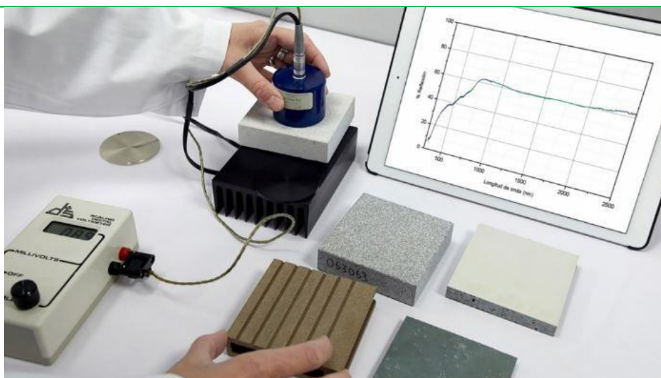
Figura.- Proceso de ensayo para determinación de SRI. Fuente [+]
