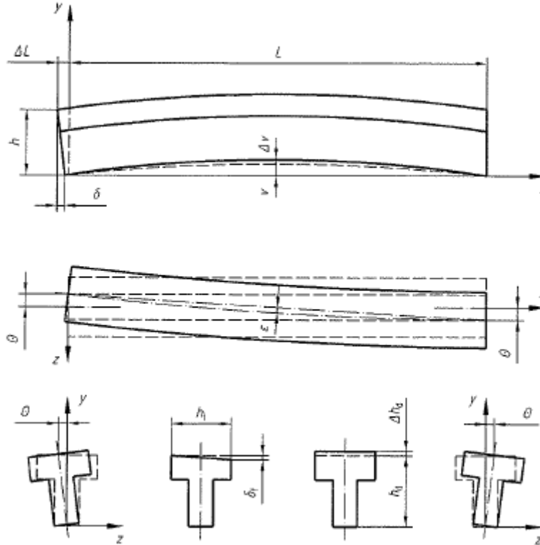
Tolerancias de las vigas
