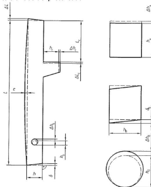
Tolerancias de las columnas
