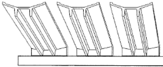
B.3a – Elementos con dos nervios simples
