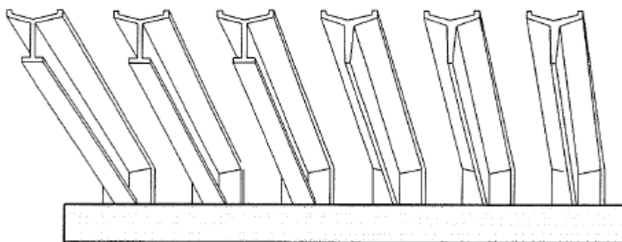
Fig. B.8 – Elementos en forma de “Y”
