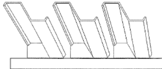
B.6c – Elementos de placa plegada en vertical
